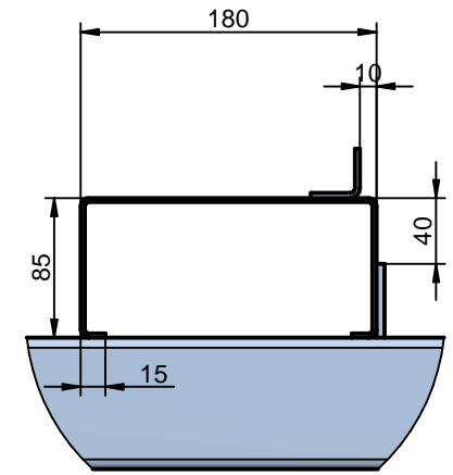
Szczegół A
